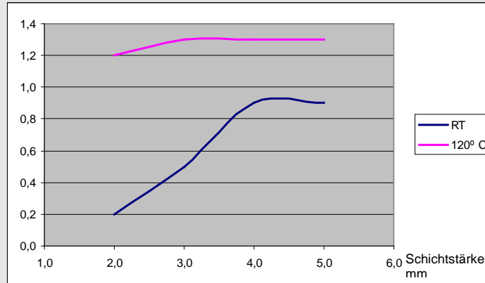
Linearer Schwund mm/m
